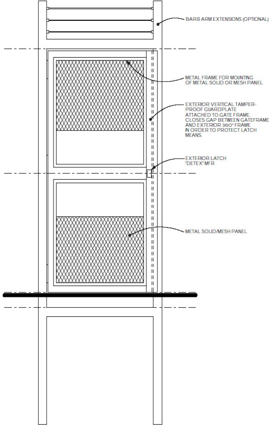
REAR ELEVATION SCALE: 1" = 1'-0"
